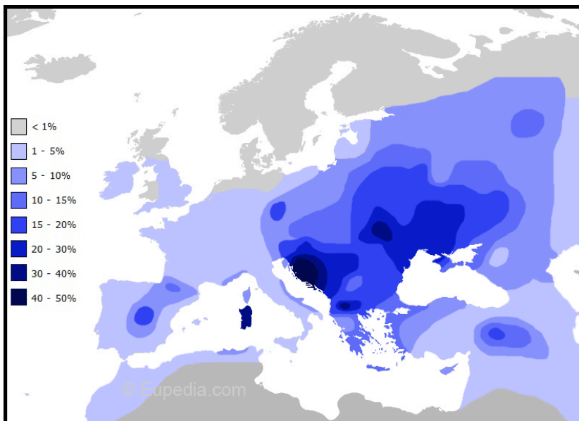
Karta 1. Starosedelačka I2a haplogrupa (MAPA I2a 1 P37.2) preuzeta sa navedenog sajta (14. 09. 2016): dnk.poreklo.rs/y-dnk-haplogrupa-i-najčešća-kod-Srba
